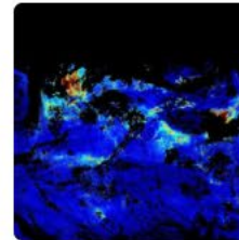
Sentinel-5p
